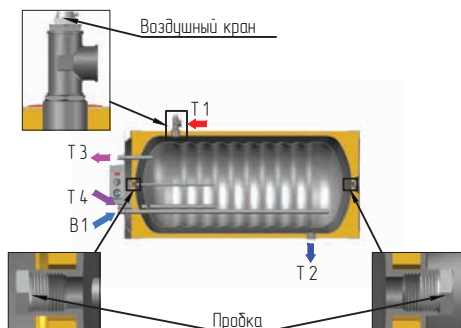
Рис. 7 Настенный горизонтальный монтаж
